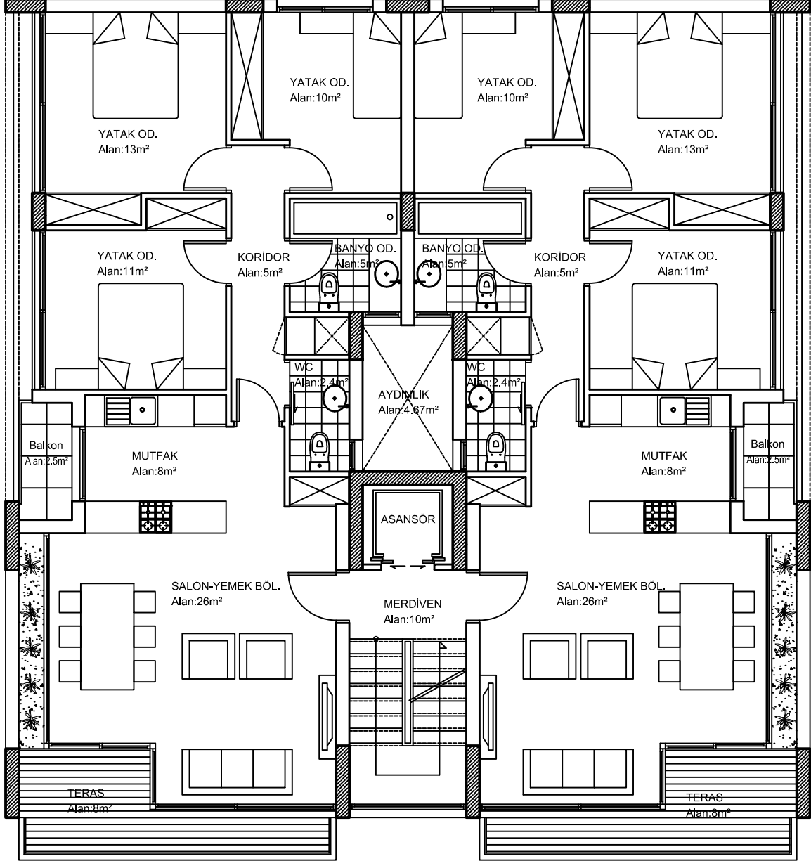
2. ve 4. KAT PLANI ÖLÇEK:1/100
